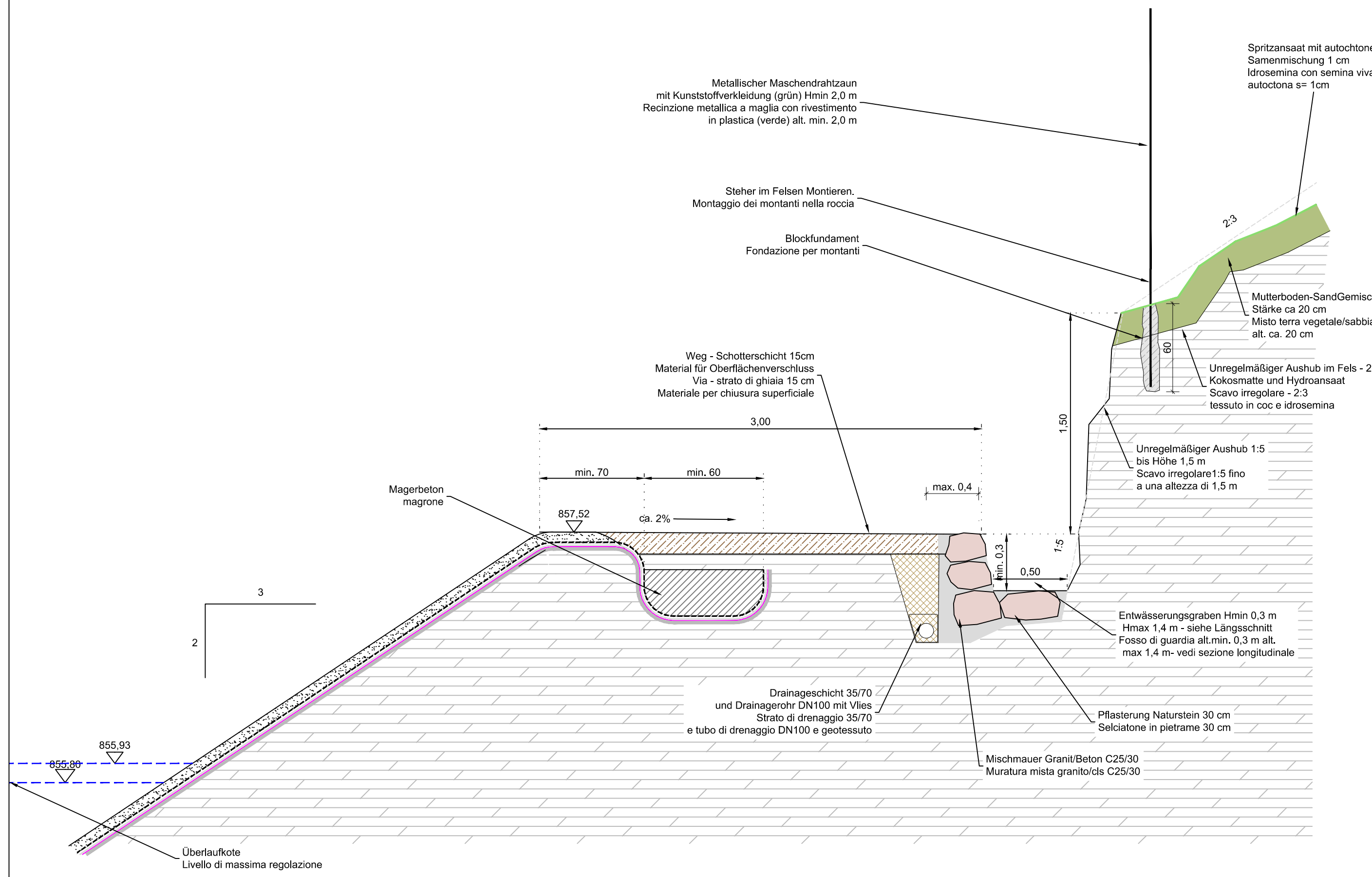
Typenschnitt Einschnitt im Fels 1:25 Sezione tipo scavo in roccia 1:25
