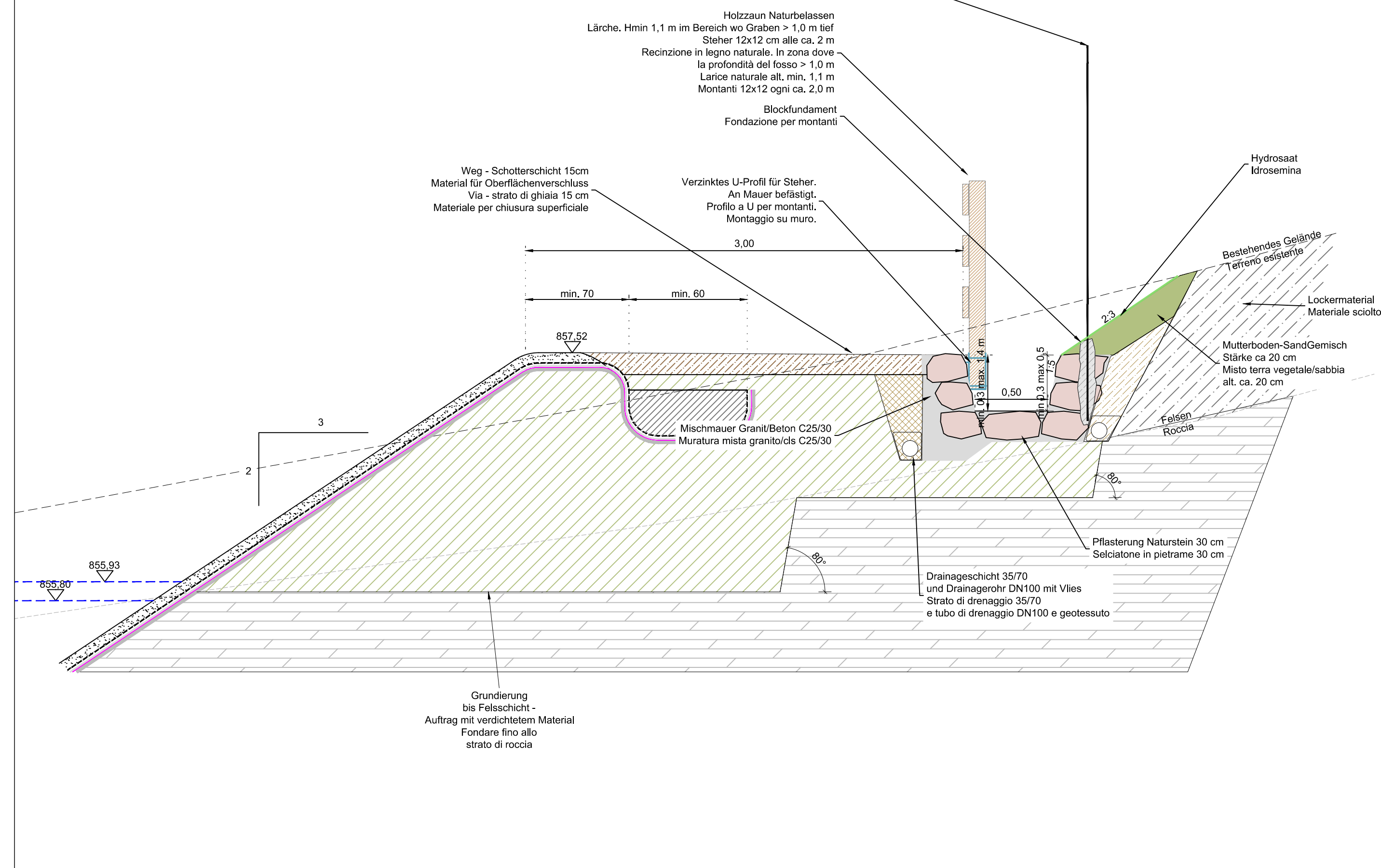
Typenschnitt Einschnitt in Lockermaterial 1:25 Sezione tipo scavo in materiale sciolto 1:25
