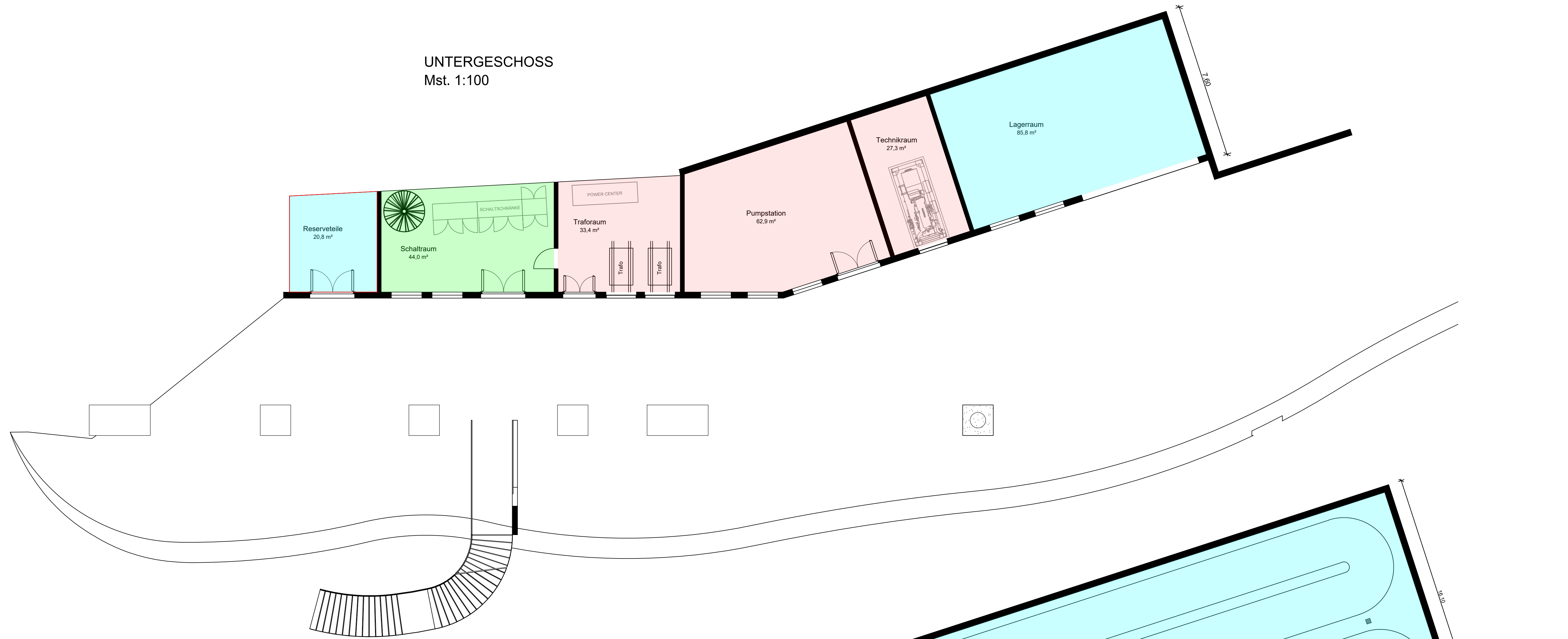
UNTERGESCHOSS Mst. 1:150
