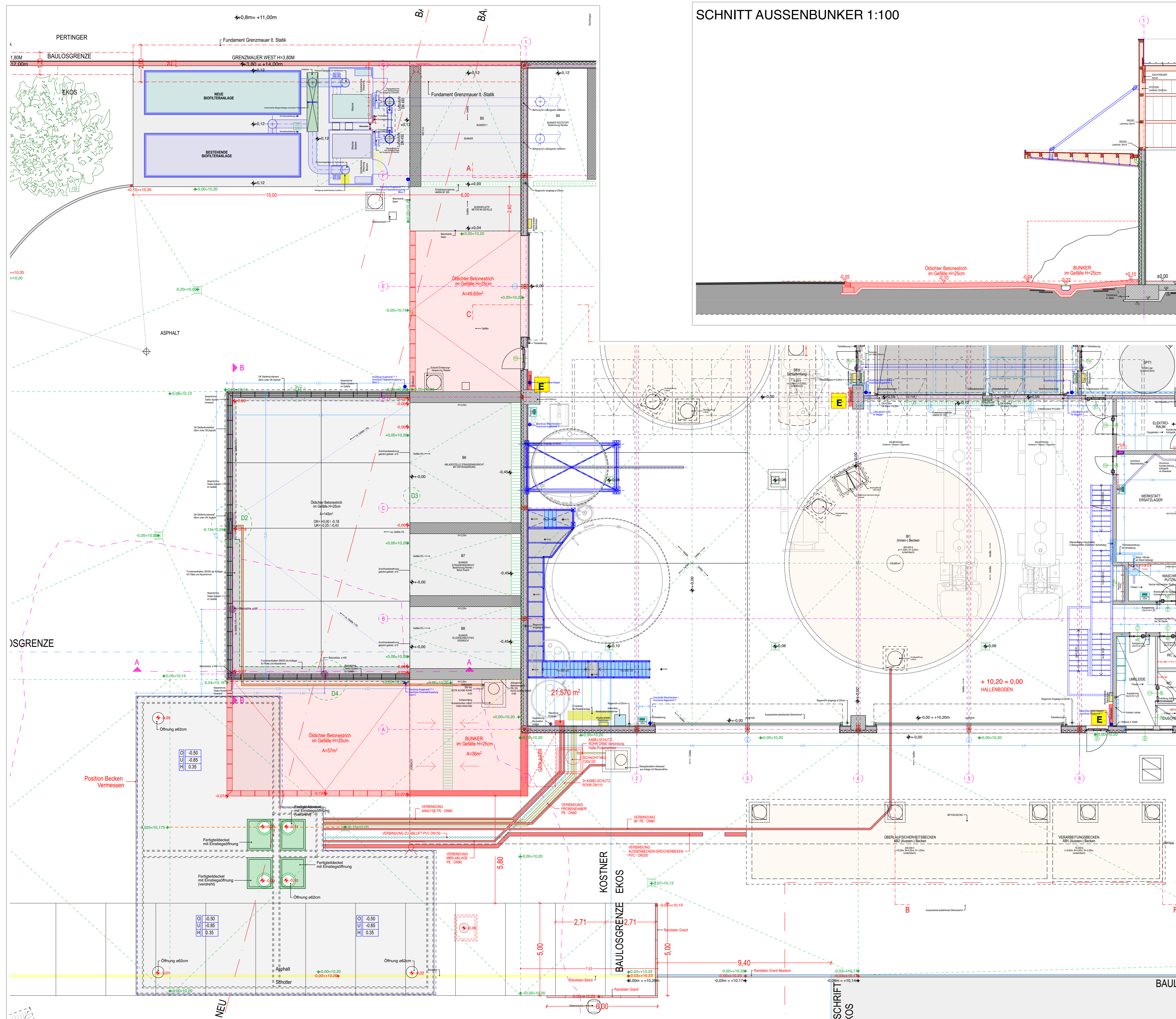
GRUNDRISS ZUSÄTZLICHER AUSSENBUNKER 1:100
