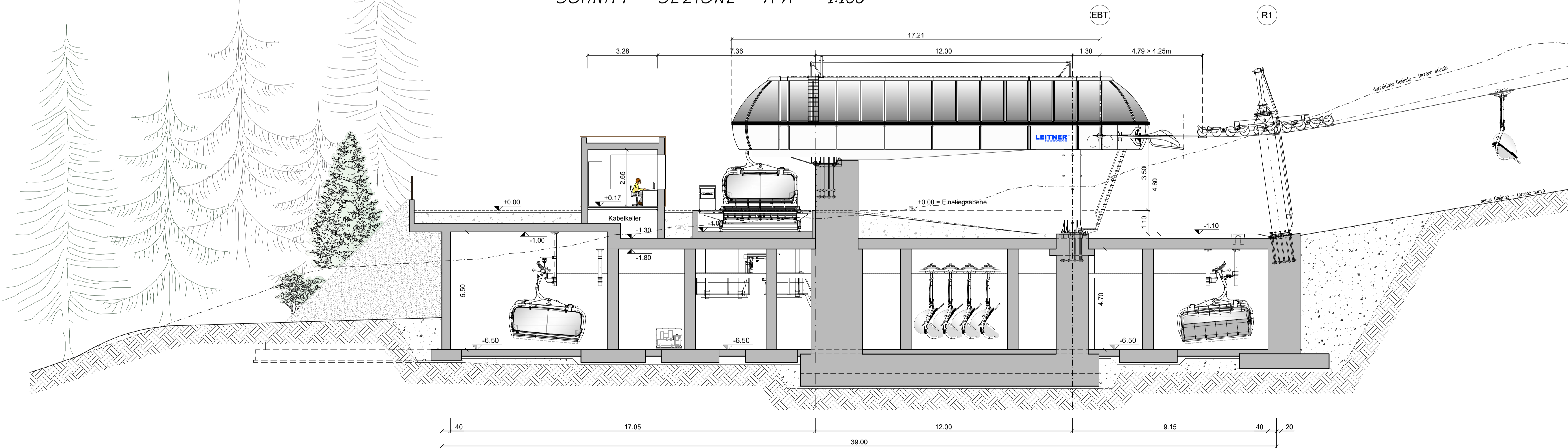
SCHNITT - SEZIONE "A-A" 1:100
